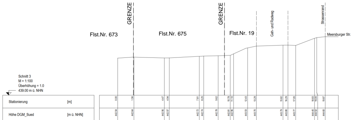
Abbildung 3a: Schnitt 3, öffentl. Parkplatz Dorfplatz, Quelle Kurzmann Maass Vermesung+Geoinformation, November 2023
